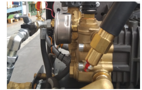
RPM decelerator kit Комплект уменьшения оборотов двигателя
